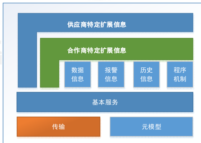
图 14 OPC UA 层模型架构
