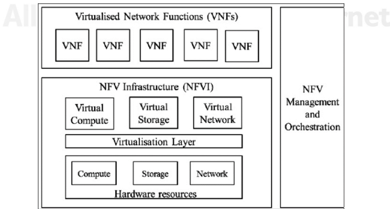
图 19 ETSI NFV 标准架构
