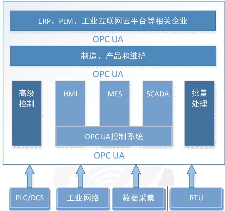
图 15 OPC UA 应用架构
