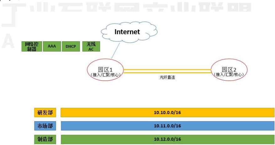
图 2 本地多园区虚拟化网络组网拓扑
