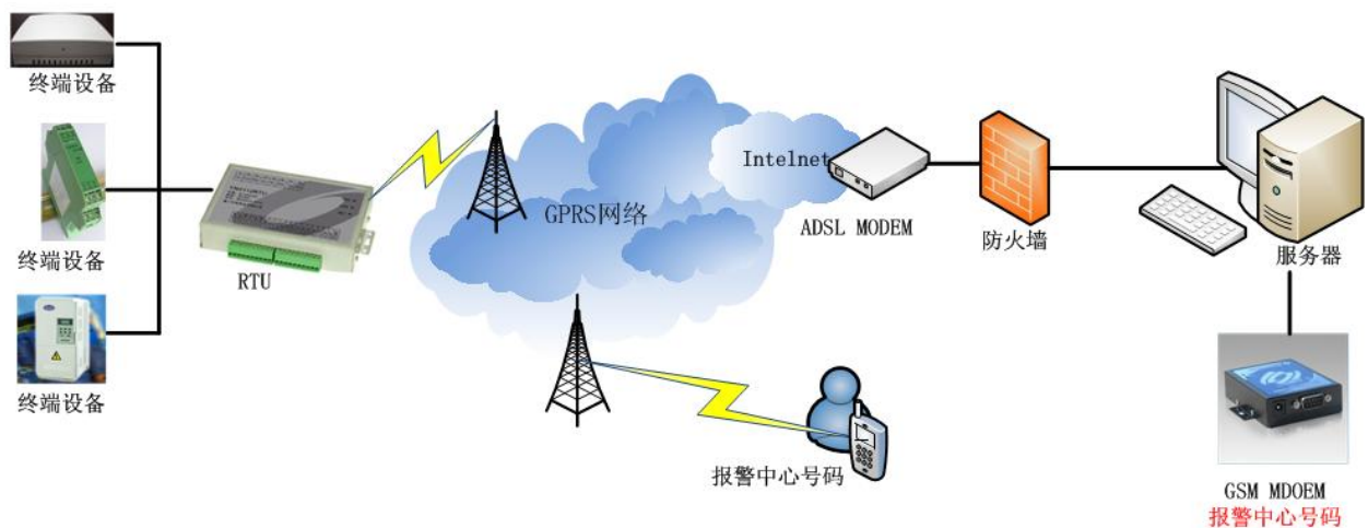
上图: YN4024-RTU 典型产品应用图框
