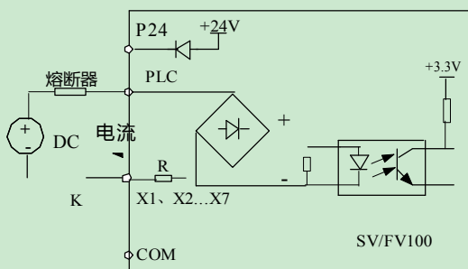
图 4-8 使用外部电源的连线方式
