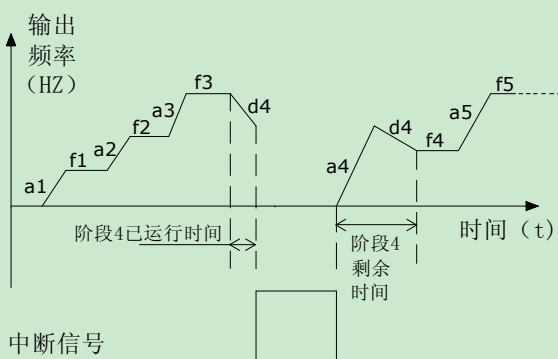
图 6-56 PLC 起动方式 2
