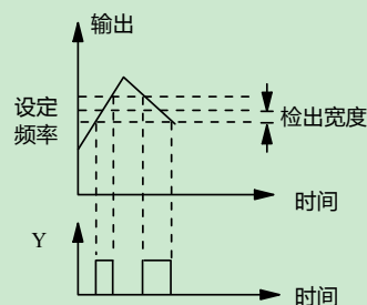
图 6-28 频率到达信号输出示意图
