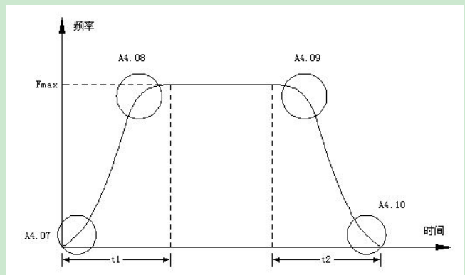
图 6-14 加减速起始、结束阶段说明
