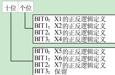
图 6-26 端子正反逻辑设定
