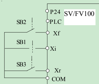
图 6-21 三线式运转模式 1
