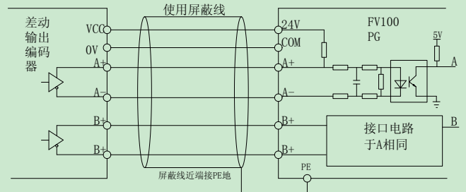
图 4-17 差分输出编码器接线图
