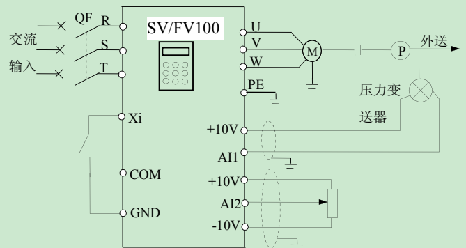
图 6-42 内置过程闭环模拟反馈控制系统示意图
