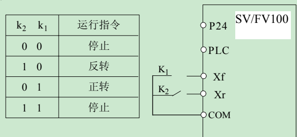
图 6-19 两线式运转模式 1
