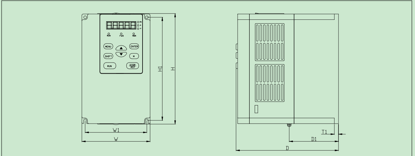
图 2-2 SV100(FV100)-4T-0037G 以下功率变频器
