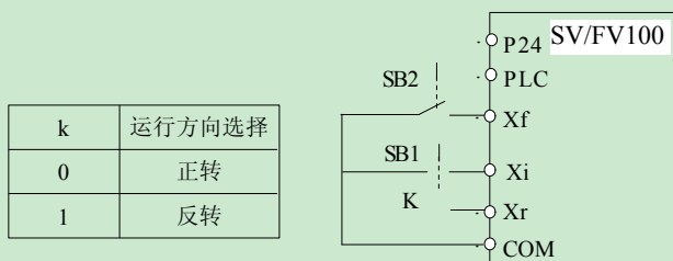
图 6-22 三线式运转模式 2
