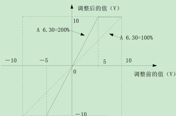
图 6-33 模拟输出与增益关系曲线
