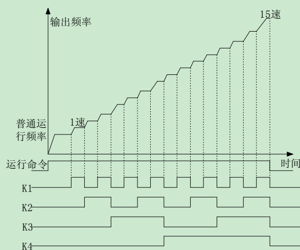
图 6-18 多段速运行示意图
