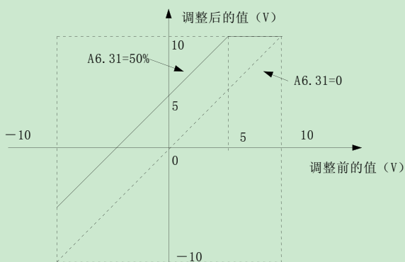
图 6-34 模拟输出与零偏关系曲线
