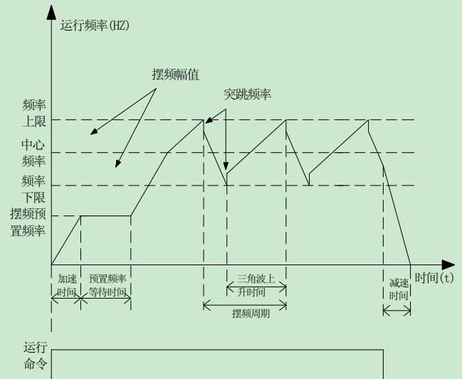
图 6-58 摆频工作示意图
