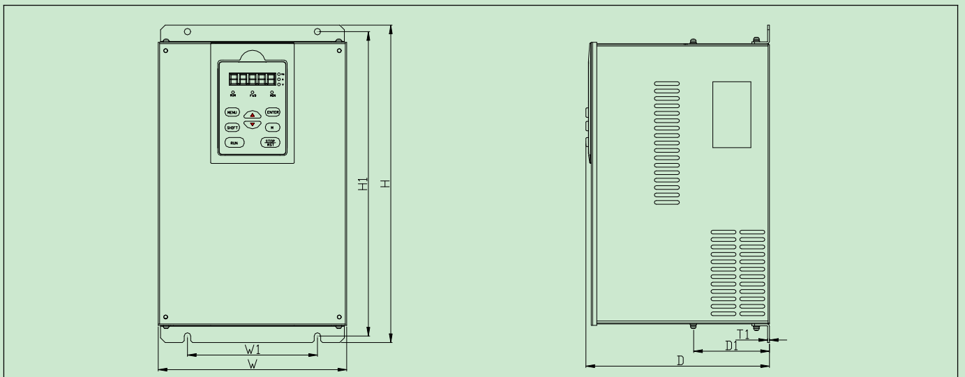
图 2-3 SV100(FV100)-4T-0055G~FV100-4T-4000G
