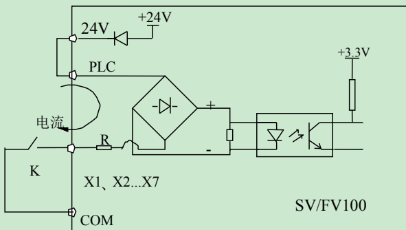
图 4-7 使用内部 24V 电源的连线方式
