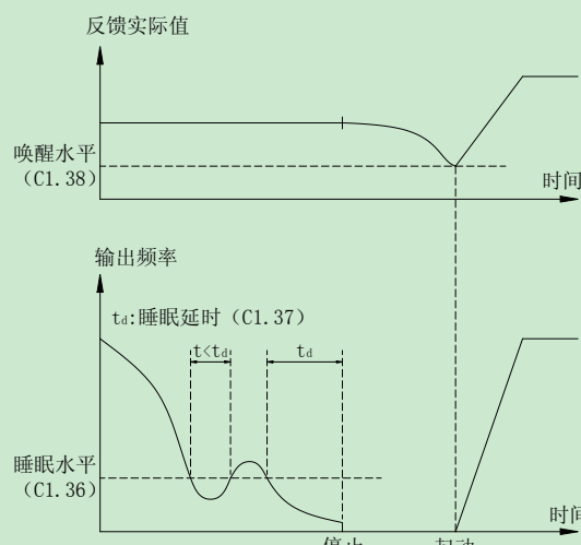
图 6-49 睡眠功能示意图
