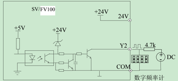
图 4-16 输出端子 Y2 连接方式 2
