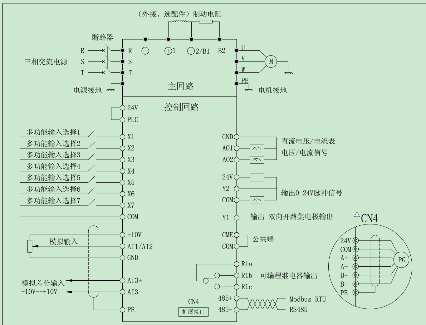
图 4-1 基本配线图
