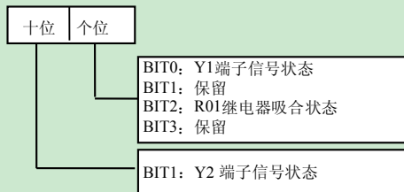
图 6-62 开关量输出状态
