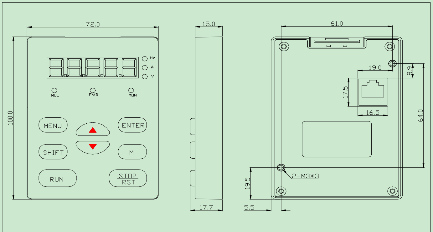
图 2-4 操作面板尺寸
