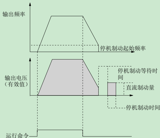
图 6-5 减速停车+直流制动示意图
