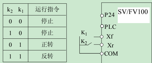
图 6-20 两线式运转模式 2
