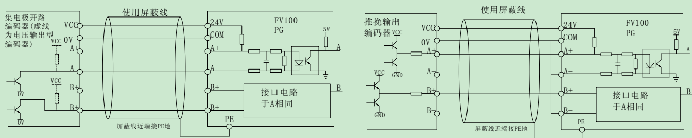
图 4-18 集电极开路编码器接线图
