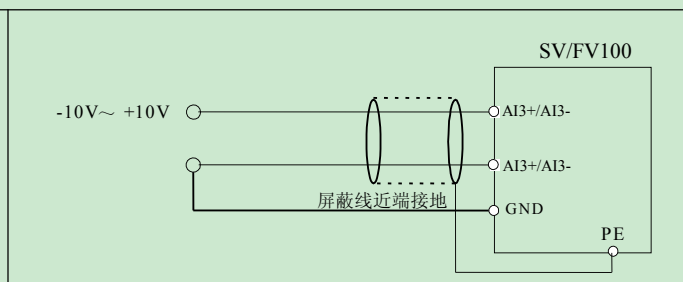
图 4-5 AI+, AI-端子单端电压输入配线图
