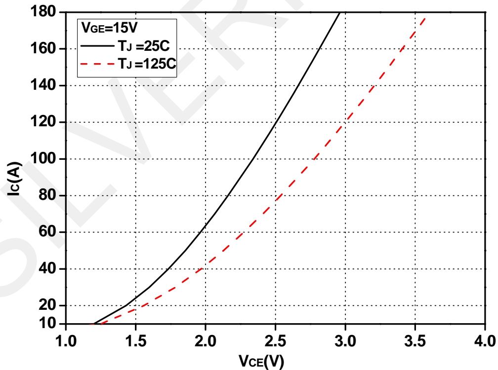
Fig.2 IGBT 电流Ic 与V CE 的典型值
