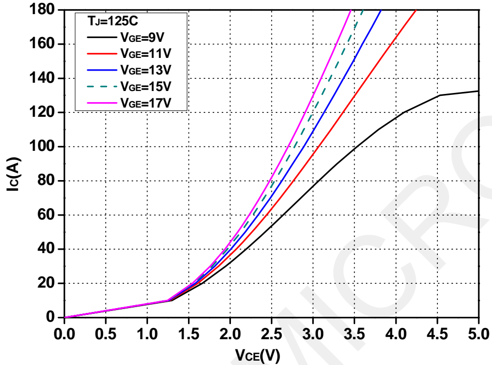
Fig.3 典型的 IGBT 输出特性
