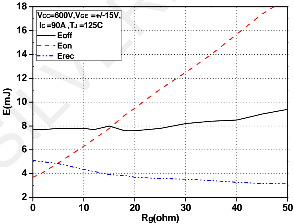
Fig.6 不同电阻时IGBT和快恢复二极管的开关损耗, T_J=125^\circ C
