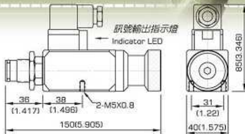
尺寸圖 / Dimension mm(inches)
