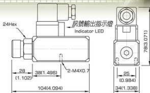
尺寸圖 / Dimension mm(inches)
