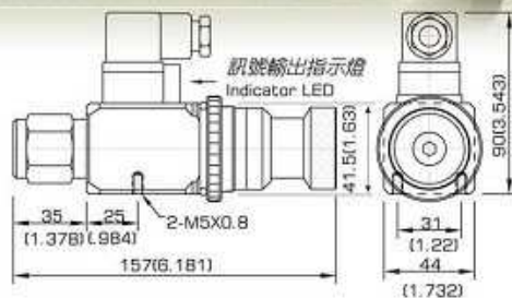
尺寸圖 / Dimension mm(inches)
