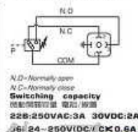
油電符號表 / Graphic Symbol
