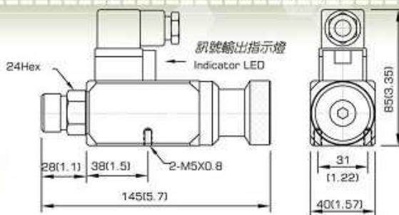
尺寸圖 / Dimension mm(inches)
