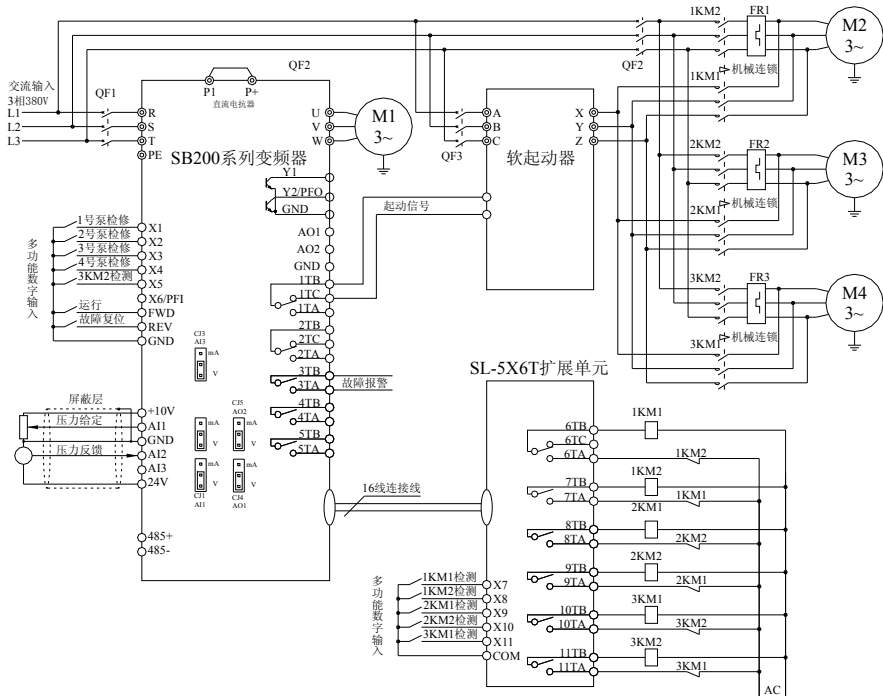
变频器加软启动器恒压供水应用图
