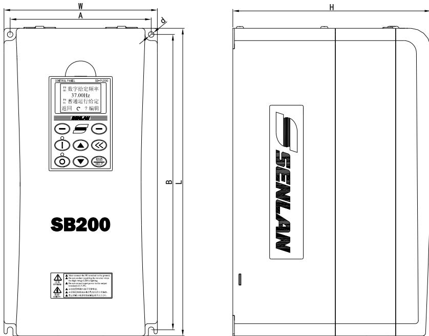
SB200-7.5T4~22T4机型外形图
