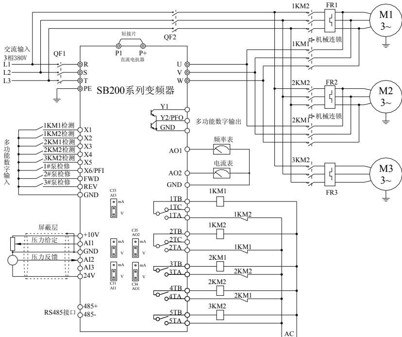
变频循环投切一控三应用图
