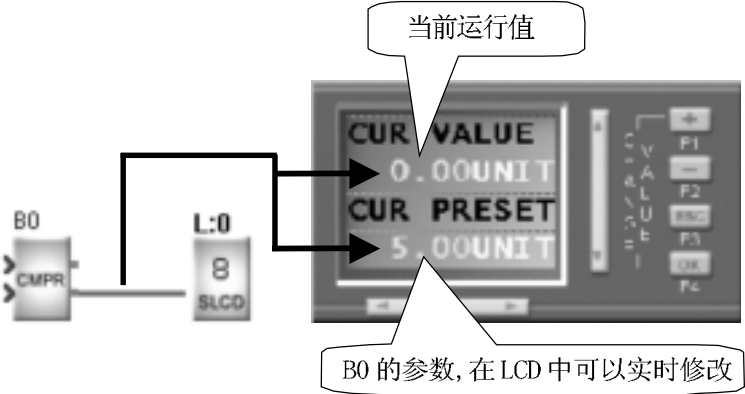
图 4.4 当前运行值及参数值
