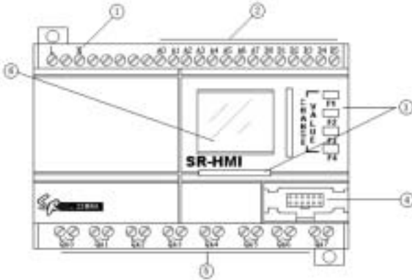
图 1.2 22 点 SR 主机系列外形图
