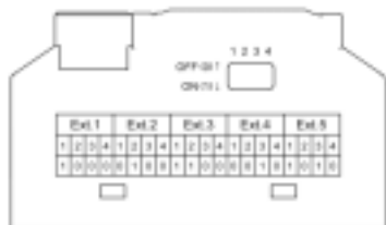
图 6.7 扩展模块地址表
