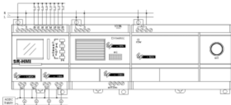
图 6.2 SR-RCA 与 SR-12MRAC、SR-VPA 的连接图
