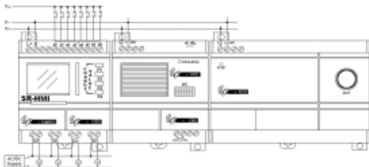
图 6.3 SR-RCD 与 SR-12MRDC、SR-VPD 的连接图
