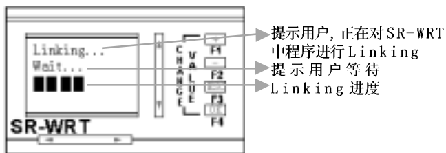
图 10.18 连接SR-WRT 的进度界面
