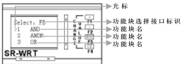
图 10.7 功能块选择界面
