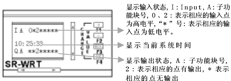
图 10.2 SR-WRT 主界面
