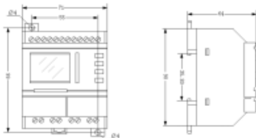
图 2.2 SR-12 系列安装尺寸 (mm)
