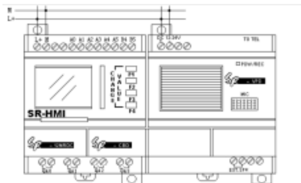
图 5.3 SR-12MRDC 与 SR-VPD 的连接图
