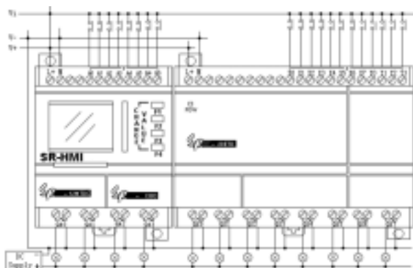
图 6.10-1 SR-20ETD 与 SR-12MTDC 接线图
