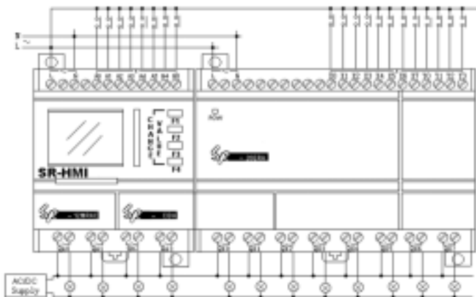
图 6.8 SR-20ERA 与 SR-12MRAC 接线图
