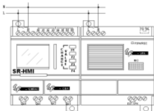
图 5.2 SR-12MRAC 与 SR-VPA 连接图
