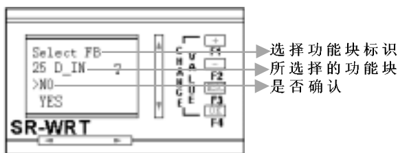
图 10.8 功能块确认界面
