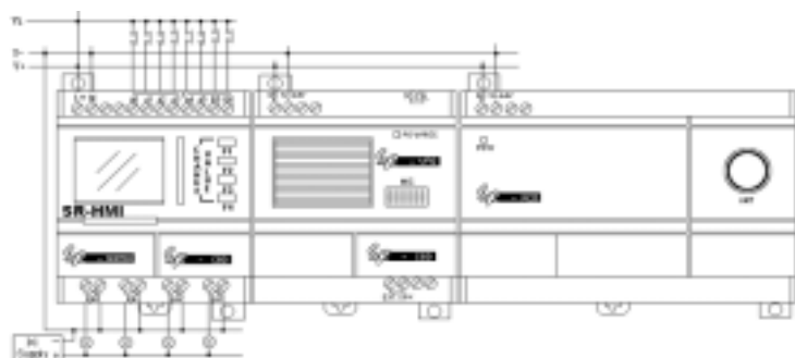
图 6.4-1 SR-RCD 与 SR-12MTDC、SR-VPD 的连接图
