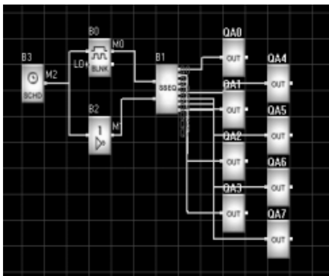
图 10.29 喷泉控制功能图
