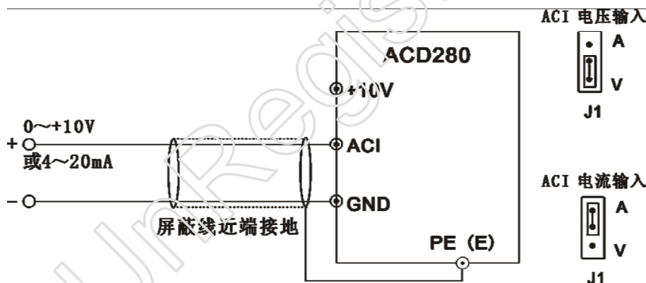
图 3-9 模拟输出端子配线
