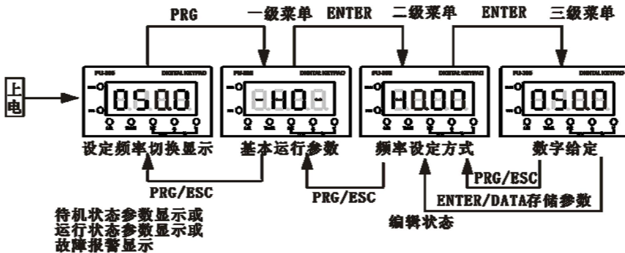
图 4-5 操作键盘显示状态的切换
