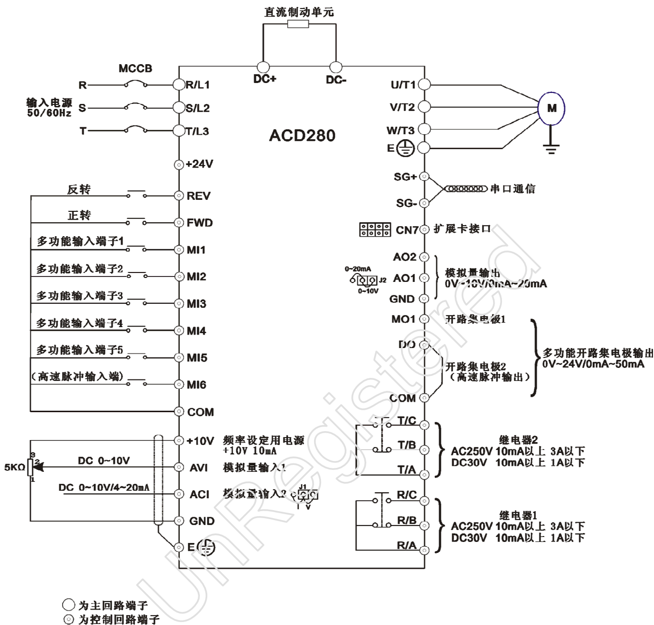
图 3-6 基本配线图
