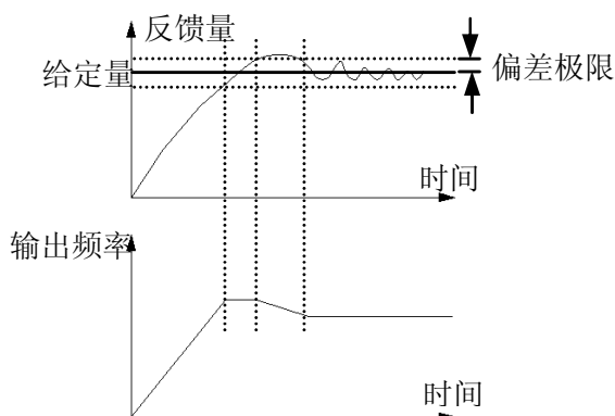
图 6-22 偏差极限示意图
