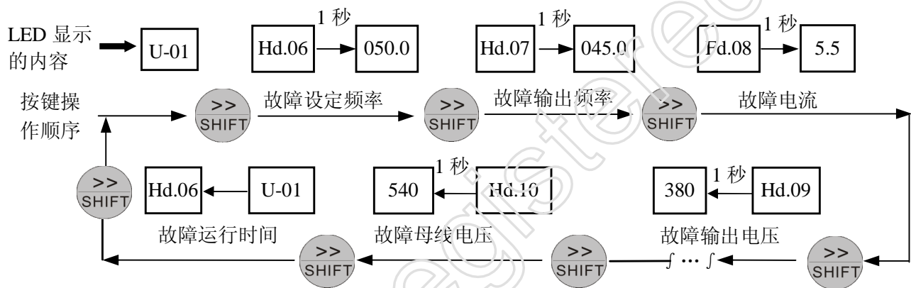
图 4-11 故障状态查询操作示例
