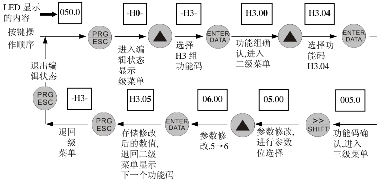
图 4-7 参数设置与修改的操作示例
