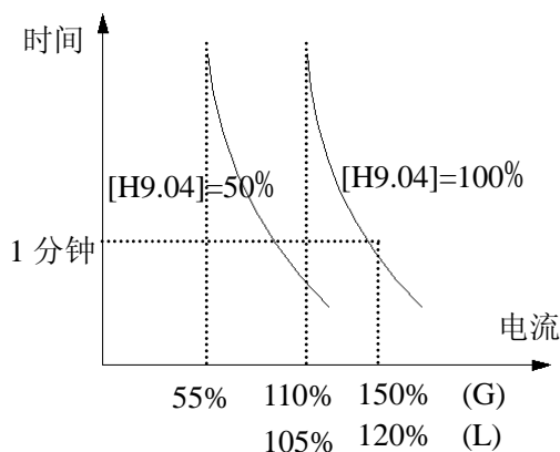
图 6-36 电子热继电器保护
