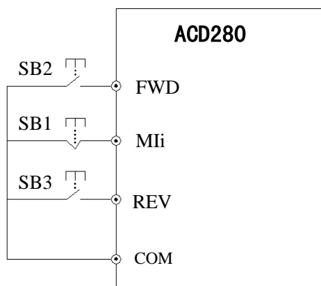
图 6-29 三线式运转模式 1
