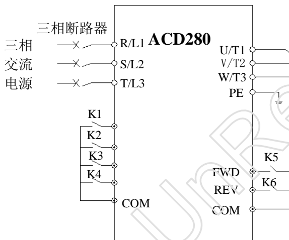
图 6-25 多段速运行接线图
