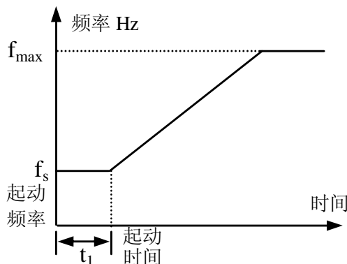
图 6-7 起动频率与起动时间示意图
