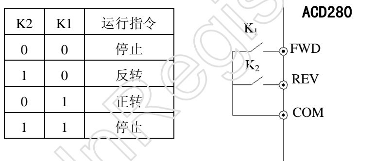
图 6-27 两线式运转模式 1
