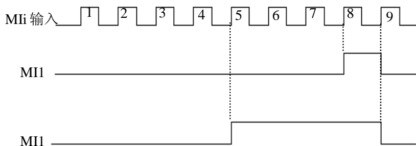
图 6-34 设定计数值给定和指定计数值给定示意图
