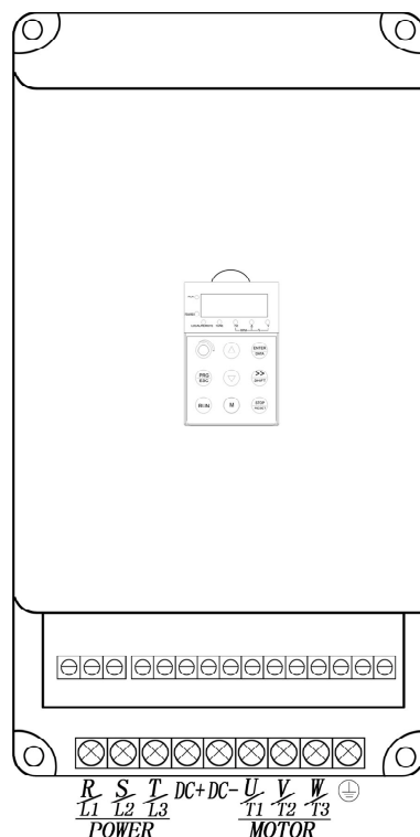
图 3-4 主回路简单配线
