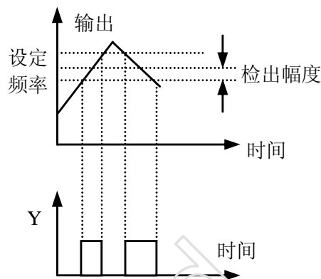
图 6-32 频率到达信号输出示意图
