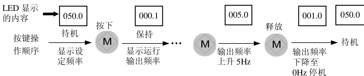
图 4-9 点动运行操作示例
