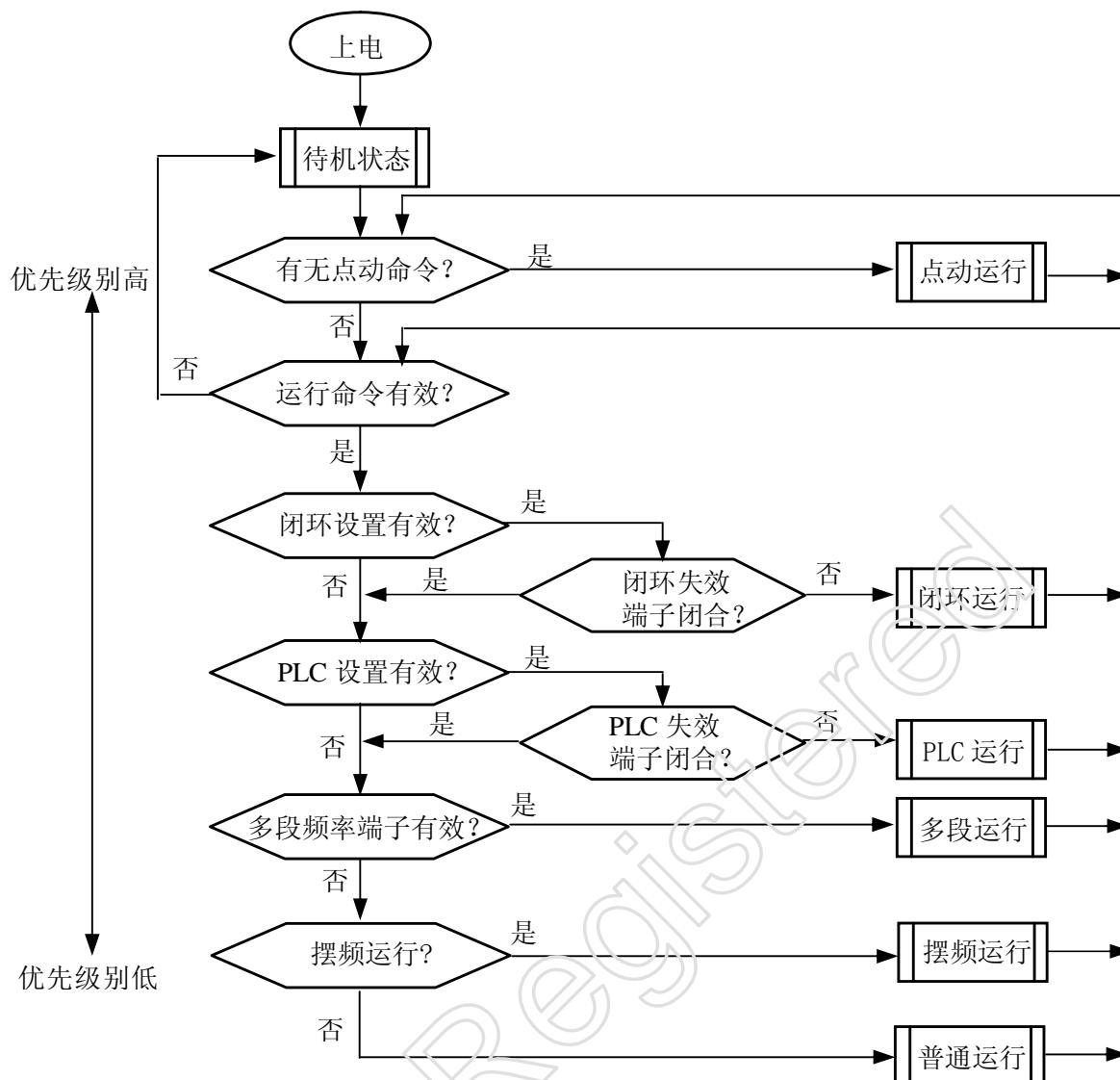
图 4-1 ACD280 变频器运行状态的逻辑程序
