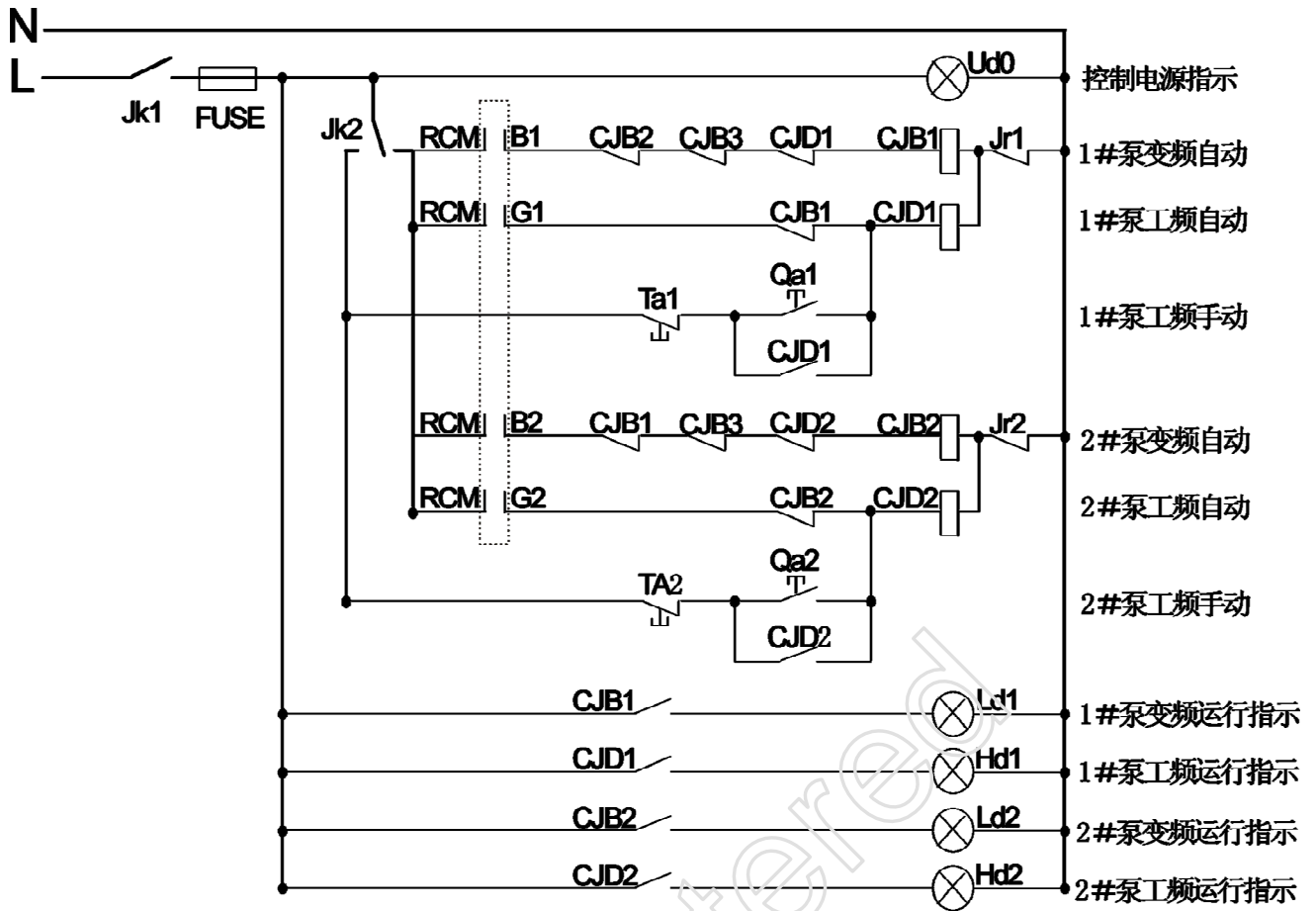
图 9-4 二次连线图
