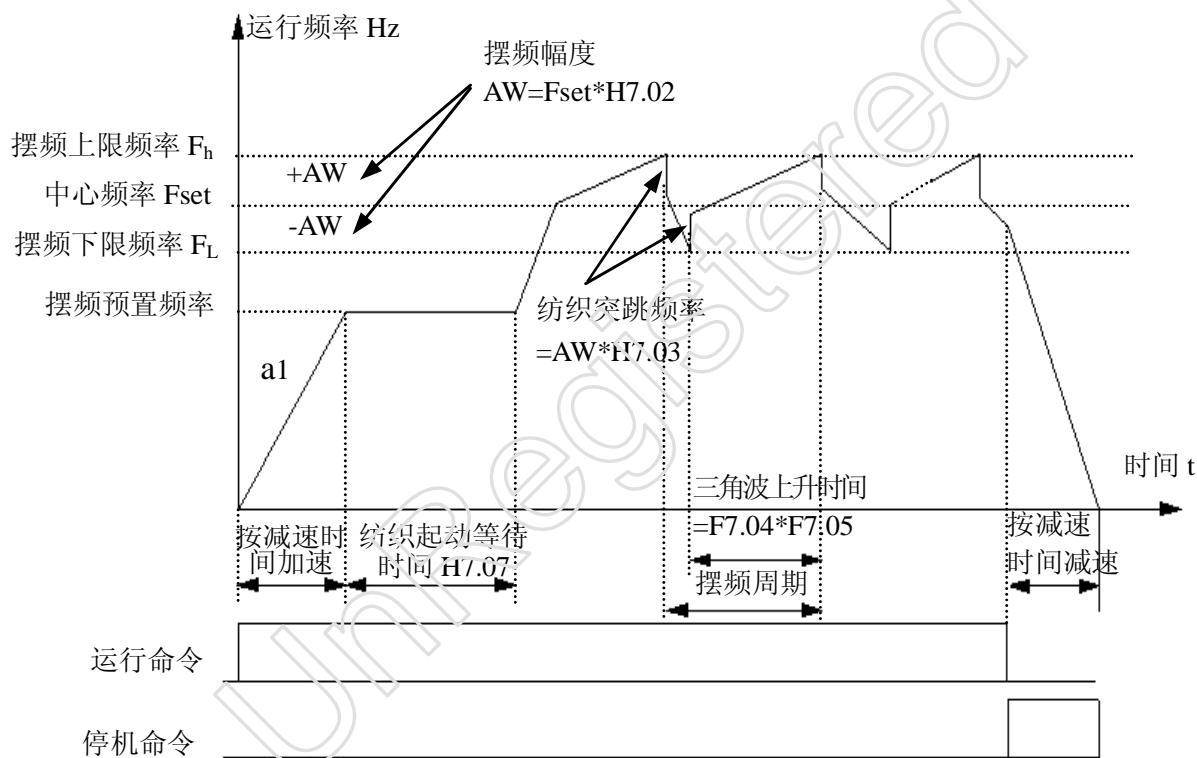
图 6-35 摆频示意图
