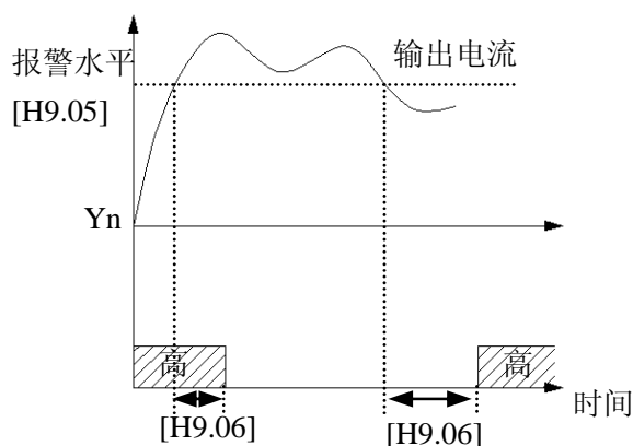
图 6-37 过载报警
