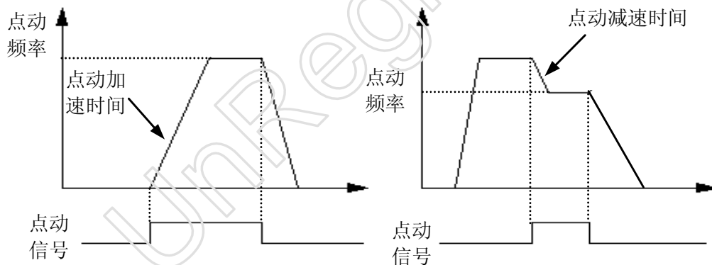
图 6-12 点动运行
