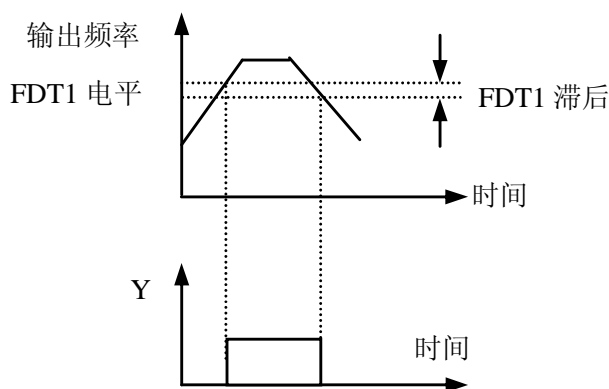
图 6-33 频率水平检测示意图
