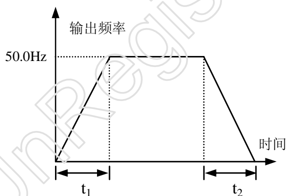
图 6-1 加减速时间定义
