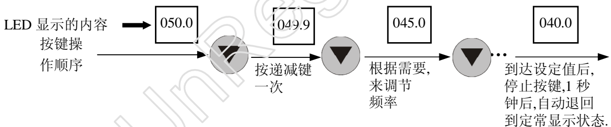
图 4-8 设定频率调整操作示例
