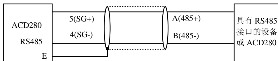
图 3-10 通讯端子配线
