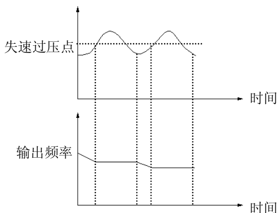
图 6-38 过压失速功能
