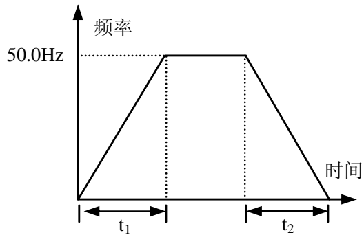
图 6-4 直线加减速
