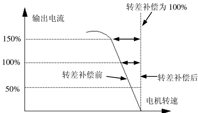
图 6-11 转差频率补偿示意图
