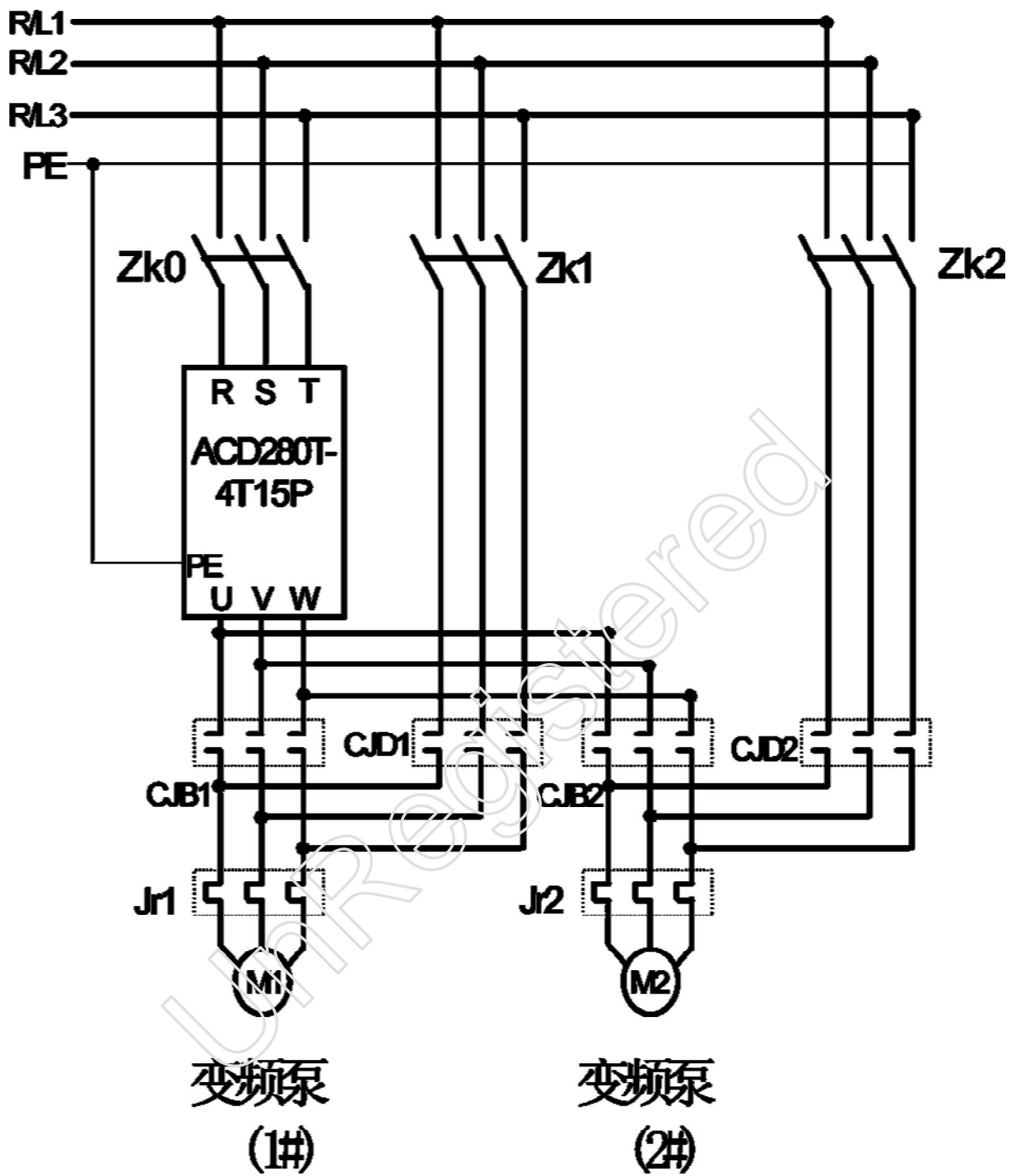
图 9-3 一次连线图
