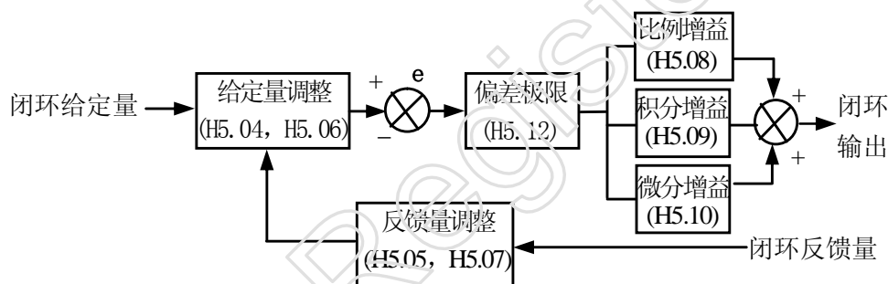
图 6-19 PID 控制原理框图
