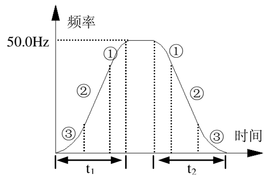
图 6-5 S 曲线加减速
