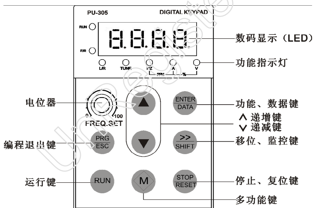
图 4-2 操作键盘布局图
