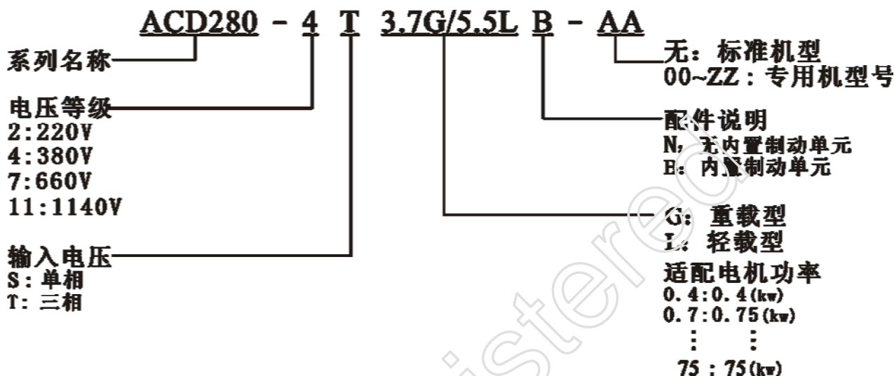
图 2-1 变频器型号说明
