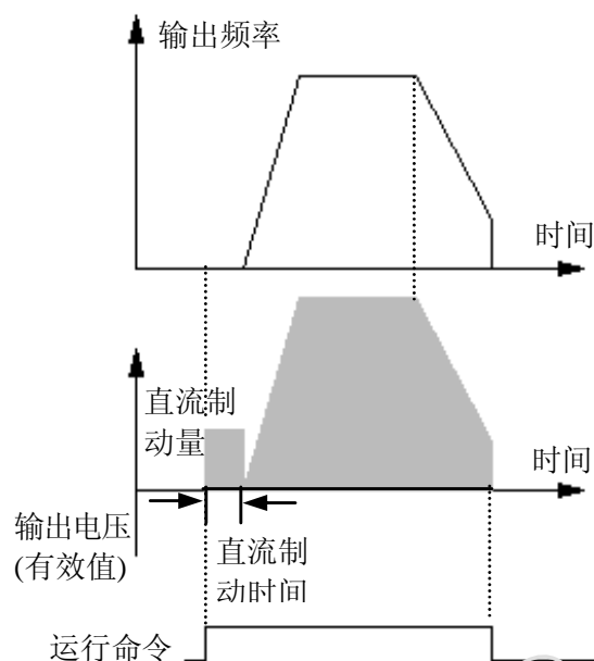
图 6-8 起动方式 1 说明
