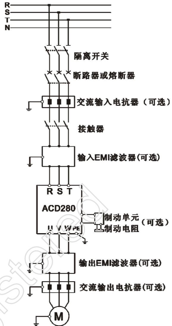
图3-5 变频器与选配件的连接
