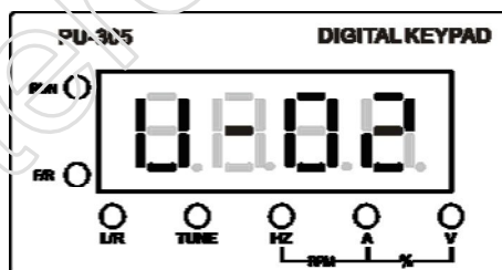
加速中过流 图 4-4 故障报警显示状态
