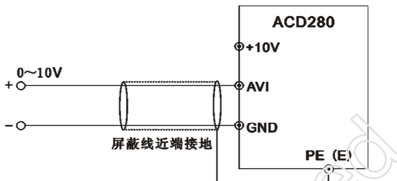
图 3-8 ACI 端子配线图
