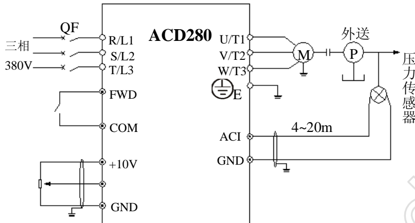
图 6-18 内置 PID 模拟反馈控制系统示意图
