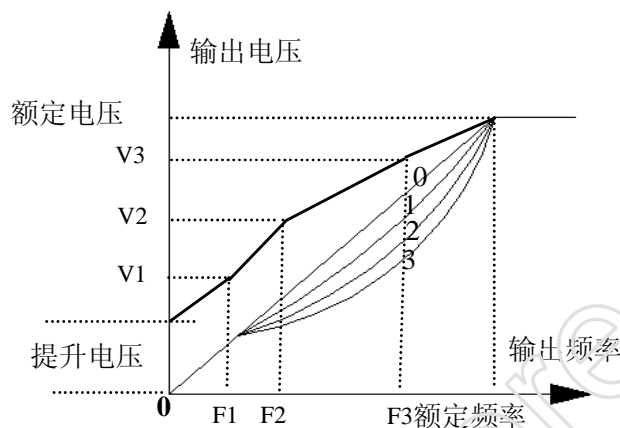
图 6-3 V/F 曲线
