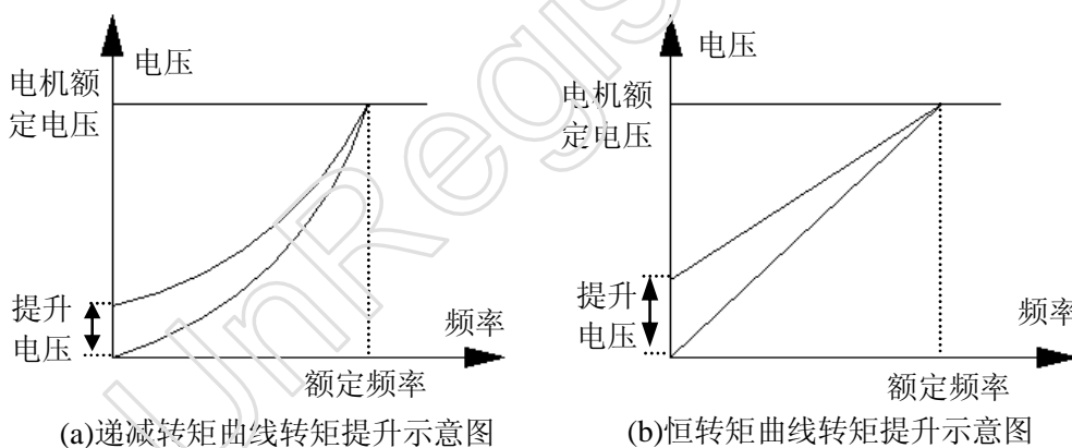
图 6-2 转矩提升示意图
