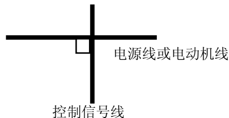
图 3-14 系统配线要求
