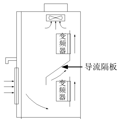
图 3-2 多台变频器的安装示意图
