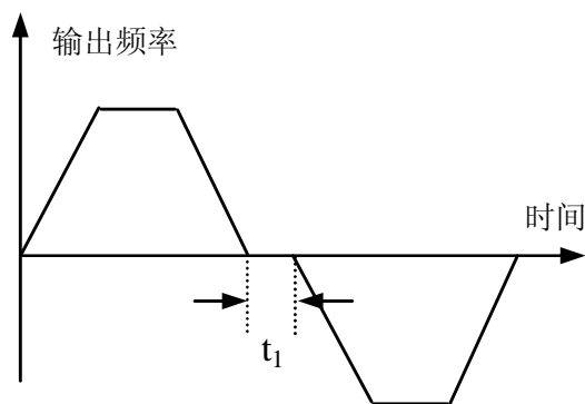
图 6-10 正反转死区时间
