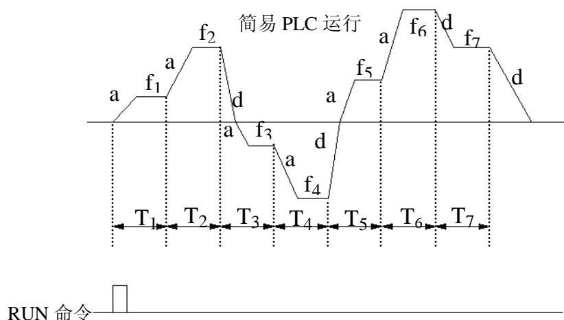
图 6-14 PLC 单循环后停机方式
