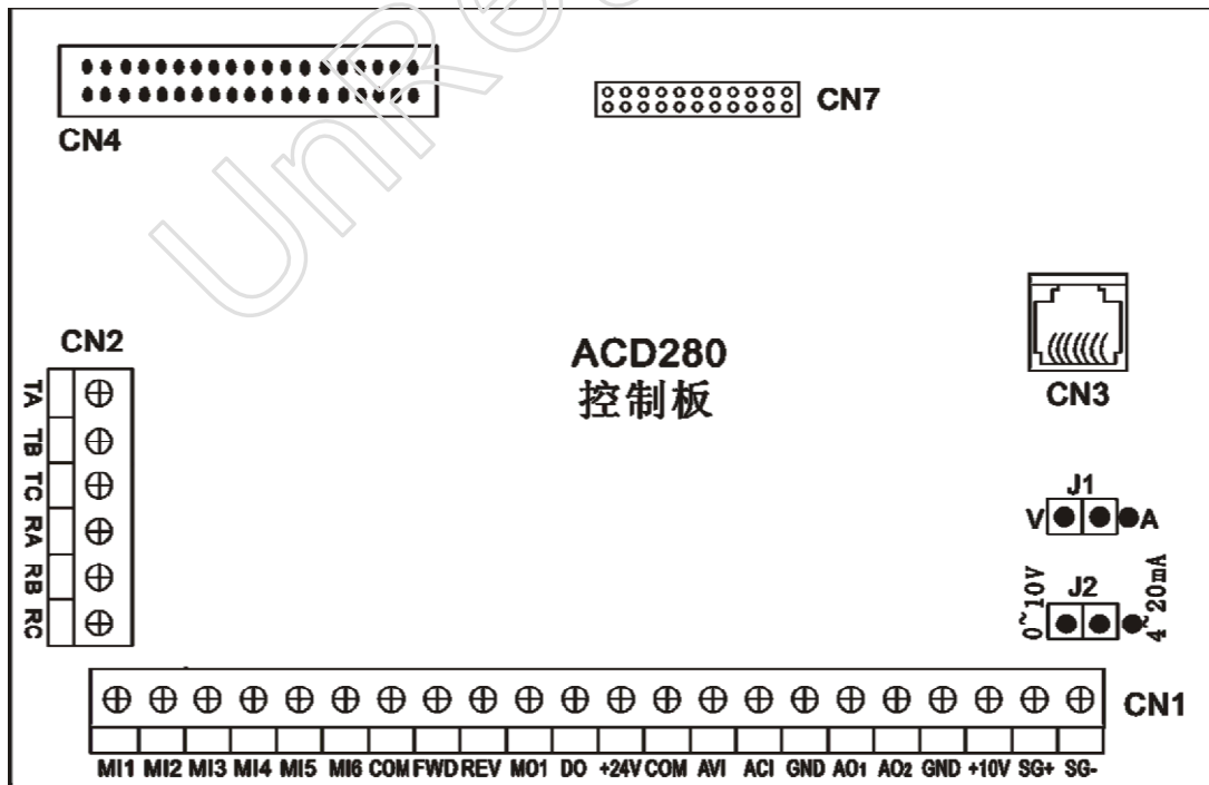
图 3-7 控制板的跳线开关位置示意图
