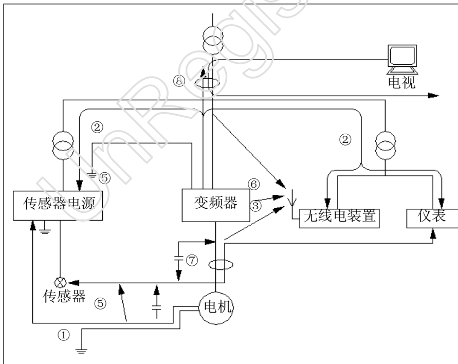
图 3-13 噪声干扰的传播路径示意图
