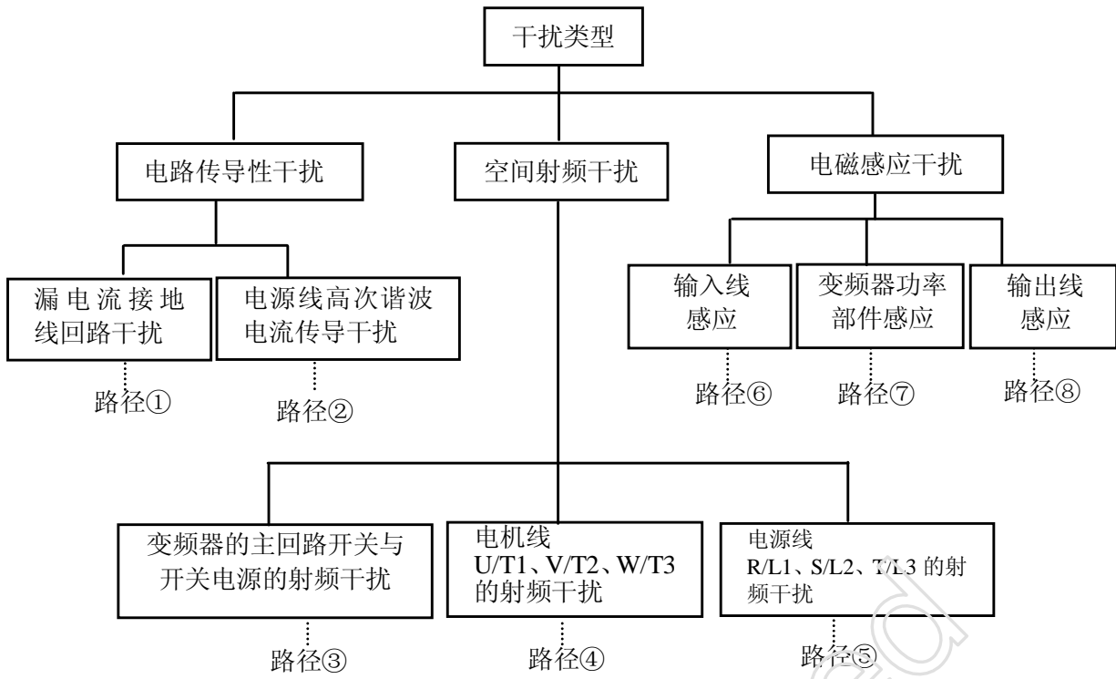
图 3-12 噪声干扰的分类
