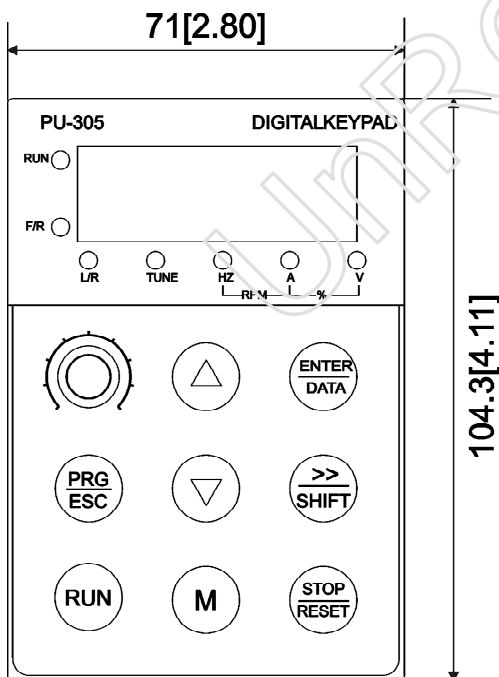
图 2-4 a 外形图
