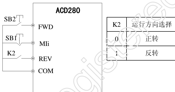
图 6-30 三线式运转模式 2
