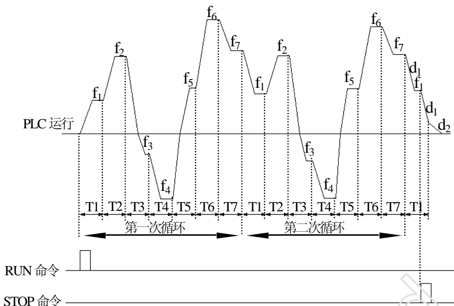
图 6-15 PLC 单循环后保持方式
