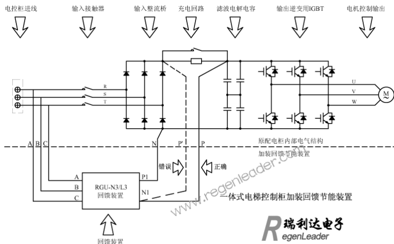
(图 3.4) RGU 系列回馈装置与电梯控制柜的连接
