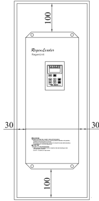
(图 3.5) RGU 系列回馈装置的安装空间要求
