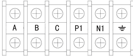
(图 3.1) RGU-N3/L3 系列回馈装置端子排列
