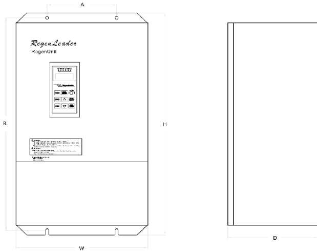
(图 2.4) RGU-F3/M3/T3 系列回馈装置的外形及尺寸
