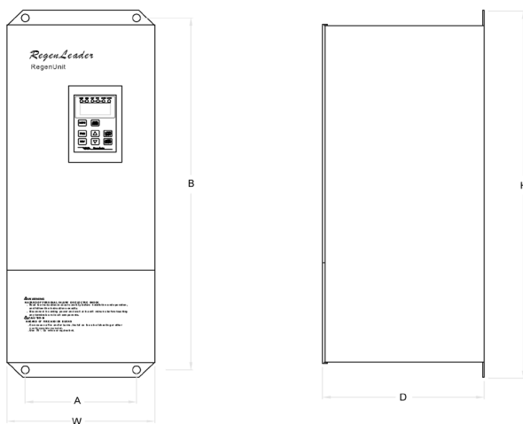
(图 2.2) RGU-N3/L3 系列回馈装置的外形尺寸
