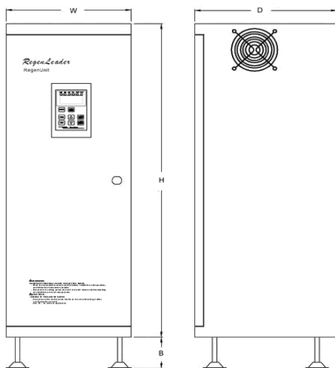
(图 2.3) RGU-LC3 系列回馈装置的外形及尺寸
