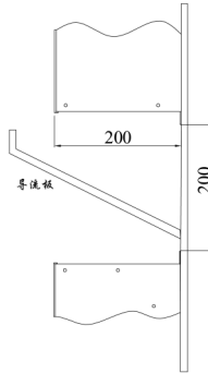
(图 3.6) 两台回馈装置上下安装示意图
