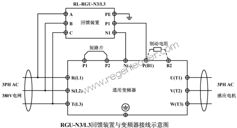
RGU-N3/L3回馈装置与变频器接线示意图
