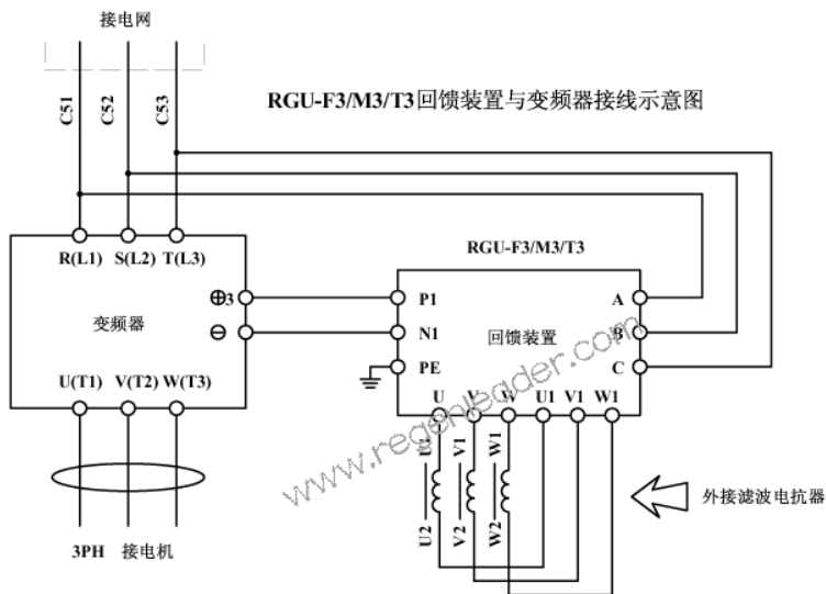
(图 3.2) RGU-F3/M3/T3 系列回馈装置与变频器的连接
